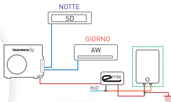
A2A MULTIZONA + ACS
