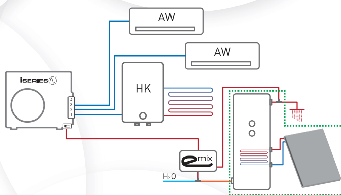
A2A + A2W + ACS + SOLARE Sistema Integrato
